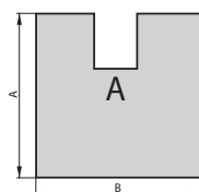
SKLO S VÝREZOM PRE CPV - FORMA „A“
