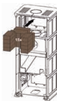
AKUMULAČNÁ SADA 94 kg (nie je súčasťou) v prípade variantu XL je potrebné objednať 2 súbavy 0424637900099
